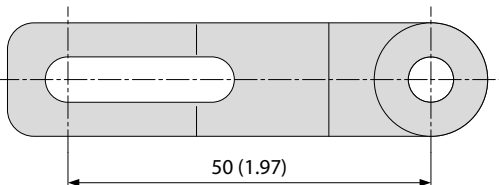
Seitenansicht: Maßstab 1:1
