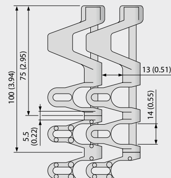
Ausführungsspezifische Abmessungen [mm (in)]
