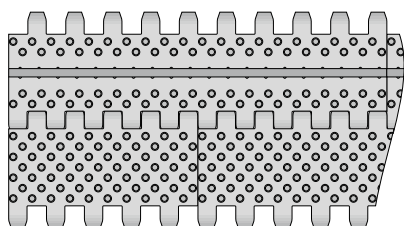
Standardanordnung S6.1-0 NCL PMU
