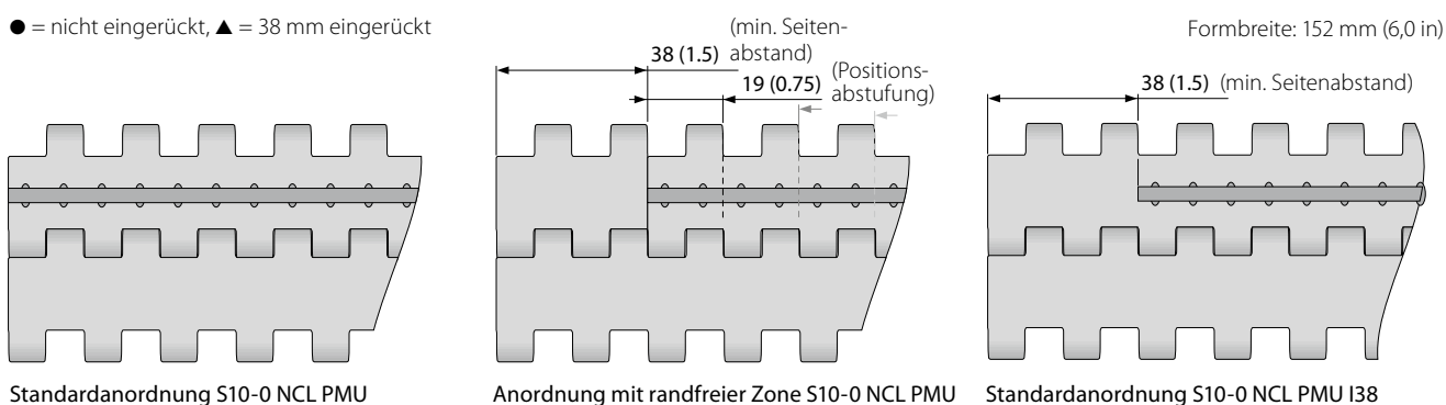
Standardanordnung S10-0 NCL PMU
