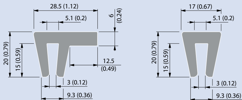
Extrudierte Gleitleisten
