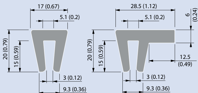
Extrudierte Gleitleisten
