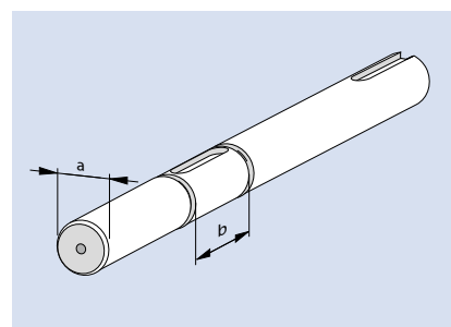
Befestigen des Zahnrads mithilfe von Sicherungsringen gemäß DIN 471 (Seegerring)
