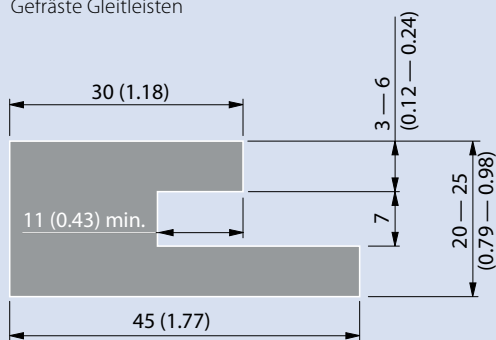
Gefräste Gleitleisten
