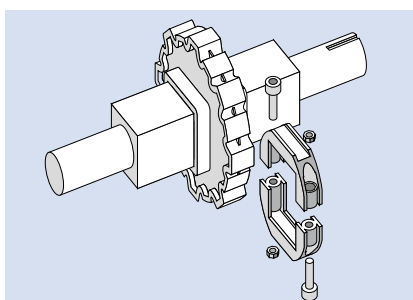
Siegling Prolink Klemmrings sind eine schnelle, einfache und zuverlässige Lösung zum Befestigen des Zahnrads (weitere Informationen dazu finden Sie auf Seite I-206 ).
