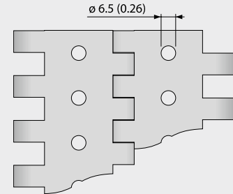
Ausführungsspezifische Abmessungen [mm (in)]
