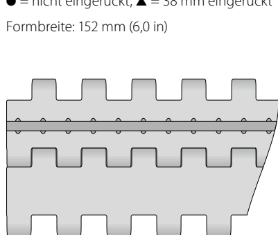
Standardanordnung S10-0 NCL PMU
