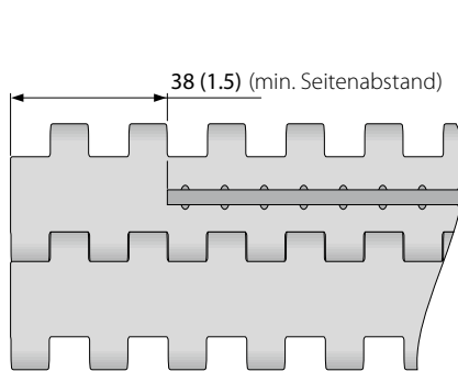
Standardanordnung S10-0 NCL PMU I38
