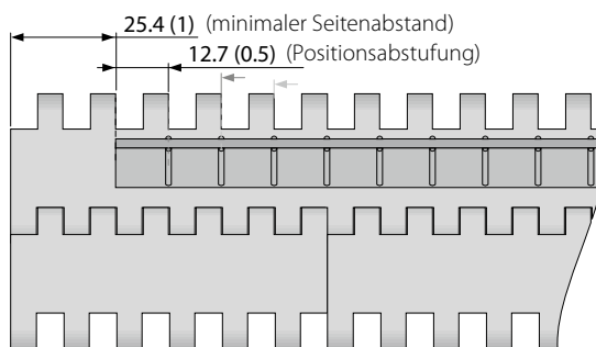
Anordnung mit randfreier Zone S8-0 FLT PMU
