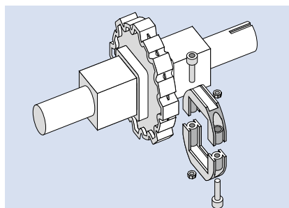
Siegling Prolink Klemmringe sind eine schnelle, einfache und zuverlässige Lösung zum Befestigen des Zahnrads (weitere Informationen dazu finden Sie auf Seite I-192 ).
