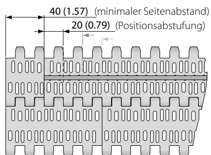
Anordnung mit randfreier Zone S6.1-23 NCL PMU
