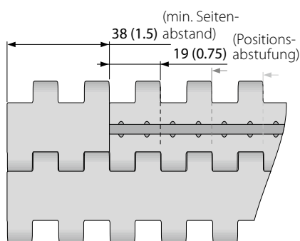
Anordnung mit randfreier Zone S10-0 NCL PMU
