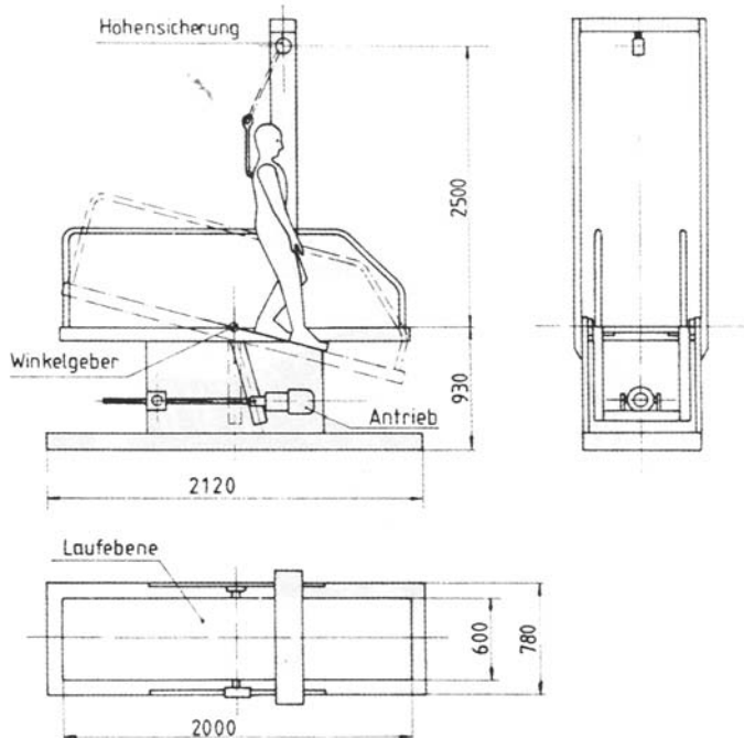
Bild 2: Prüfeinrichtung (Schiefe Ebene)
