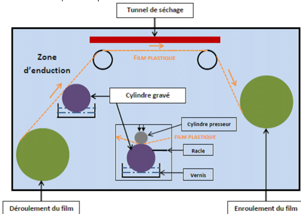
Figure 1 : Procédé d'enduction
