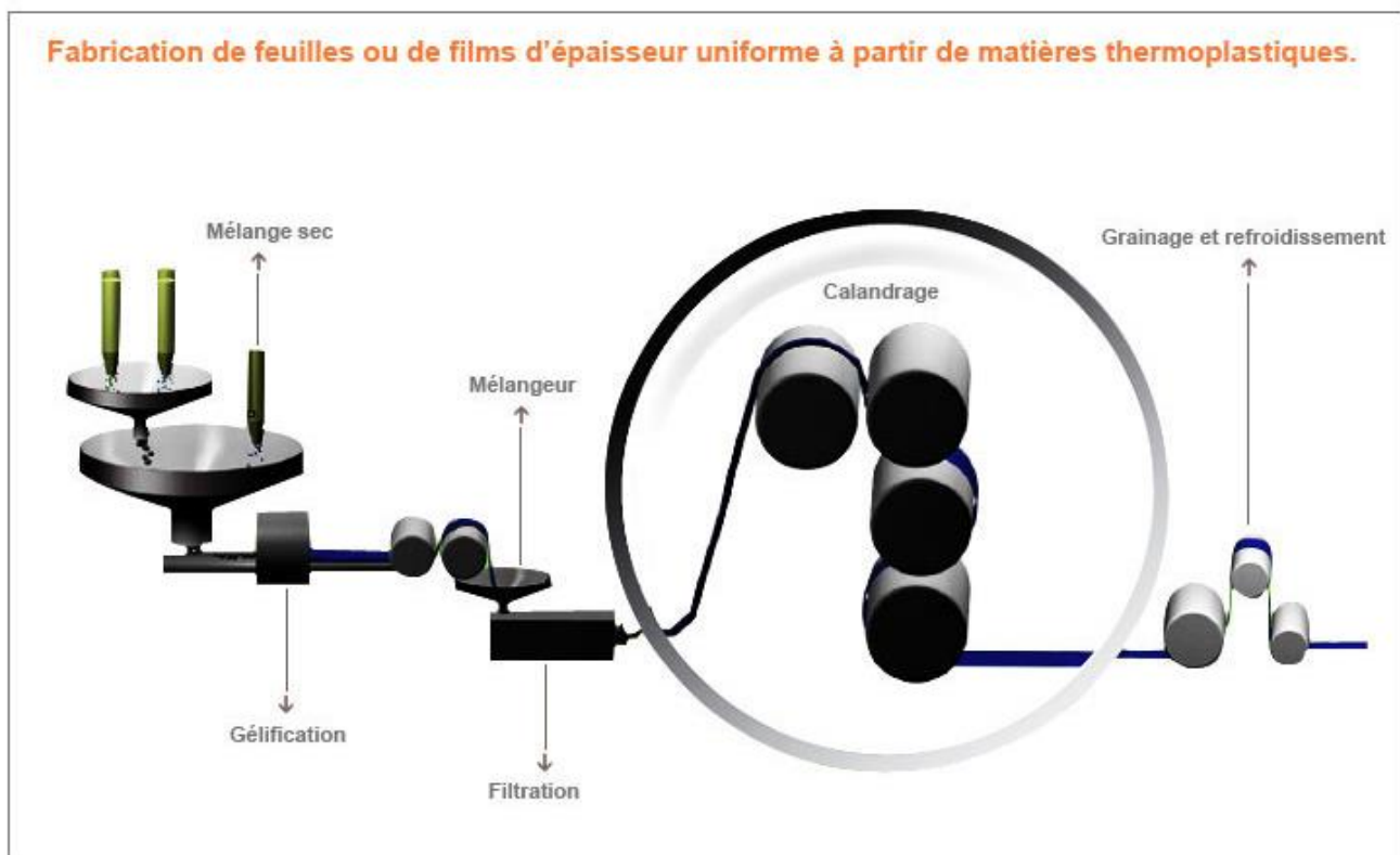
Figure 2 : Processus de calandrage
