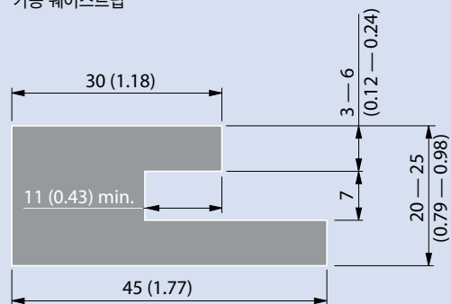
가공 웨어스트립
