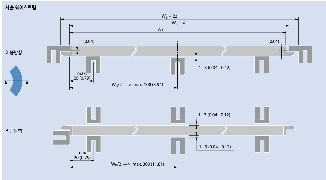
홀드 다운 캡이 부착된 시리즈 11 웨어스트립 권장 배열
