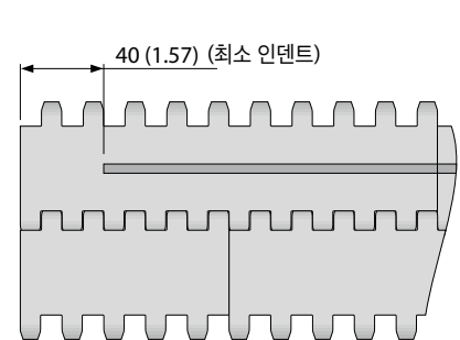
기본 배열 S6.1-0 FLT PMU I40
