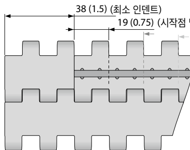
인텐트 배열 S10-0 NCL PMU
