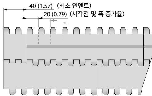
인덴트 배열 S3-0 FLT PMU
