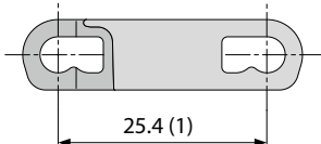
측면도 스케일 1:1
