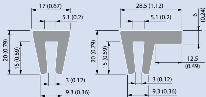
사출 웨어스트립
