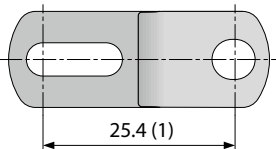
측면도 스케일 1:1
