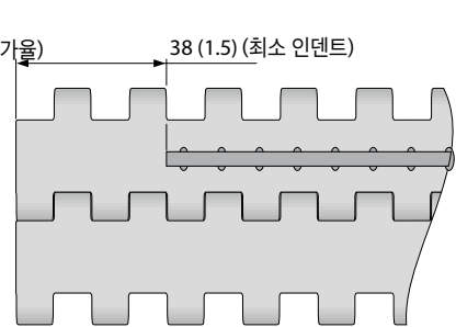
기본 배열 S10-0 NCL PMU I38
