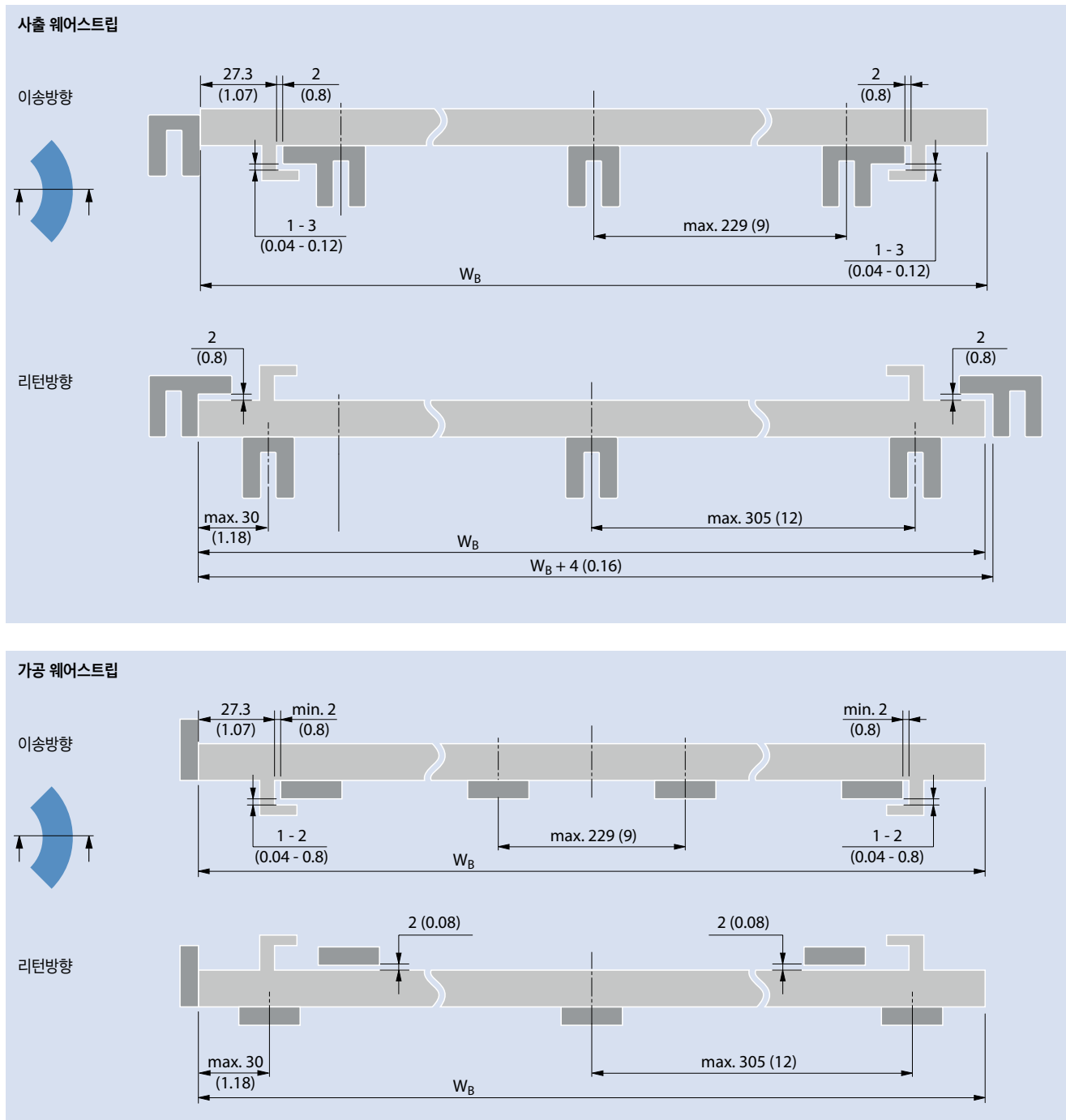
시리즈 18 변형 S18-44 GRT G 웨어스트립 권장 배열
