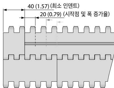
인덴트 배열 S6.1-0 FLT PMU
