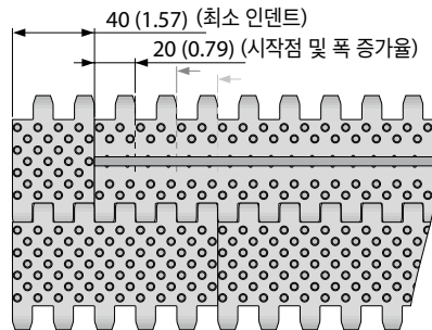
인덴트 배열 S6.1-0 NCL PMU
