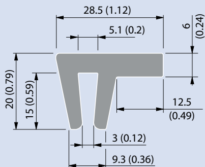
사출 웨어스트립
