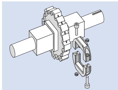
시글링 프로링크 리테이너 링은 신속, 편리, 정확하게 스프로킷 고정 솔루션을 제공( I-190 페이지 참조).
