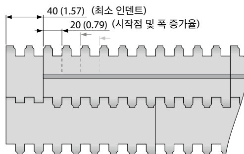
인덴트 배열 S3-O FLT PMU
