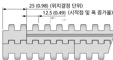
인덴트 배열 S4.1-0 FLT/NCL PMU
