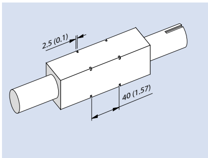
샤프트 40 x 40 mm, DIN 471 (스냅링) d=56 mm에 따라 스프로킷 체결. (세부 규격에 대해서는 부록 VI-11페이지 를 참조)
