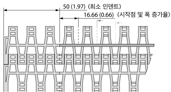
인텐트 배열 S2-57 GRT PMC
