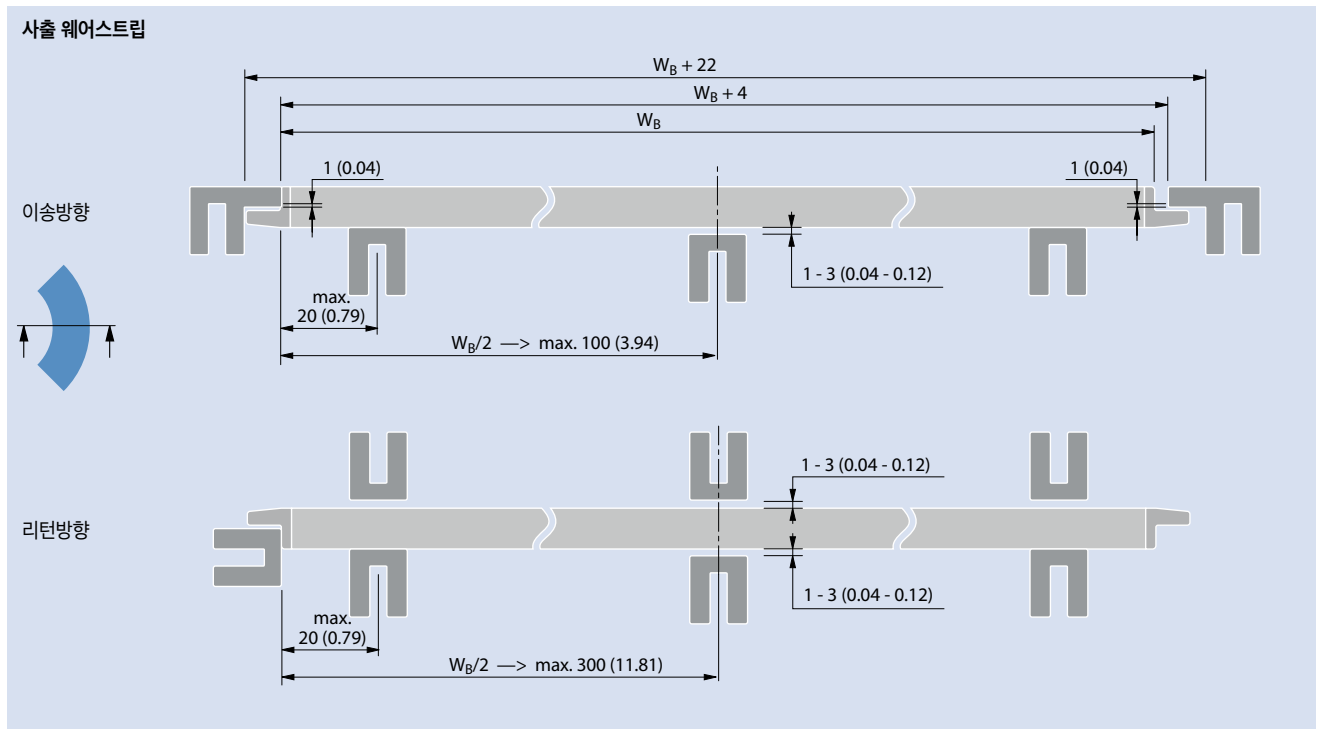
HD 캡이 부착된 S11 웨어스트립 배열
