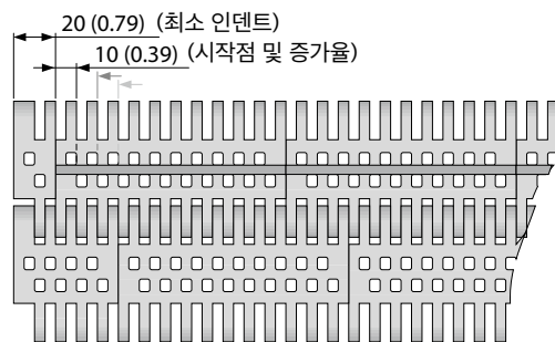
인덴트 배열 S1-18 FLT PMC
