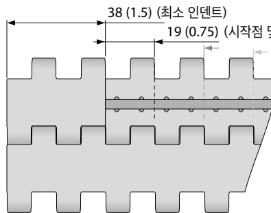
인덴트 배열 S10-0 NCL PMU
