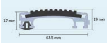
Nuway Grid 17 mm met Ultragrip Rubber
