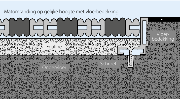
Doorsnede van een verzonken frame bevestigd met schroeven.
