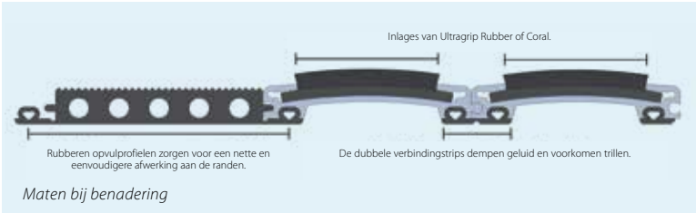
Nuway Grid 12 mm met Coral
