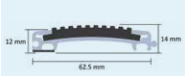
Nuway Grid 12 mm met Ultragrip Rubber
