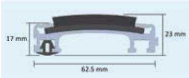
Nuway Grid 17 mm met Coral
