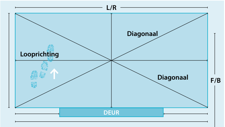
Opmeten van de uitsparing
