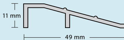
ARF 70
