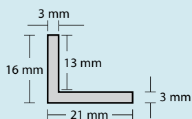
AMF 163
