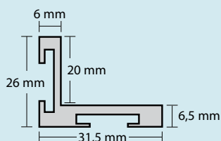
AMF 213
