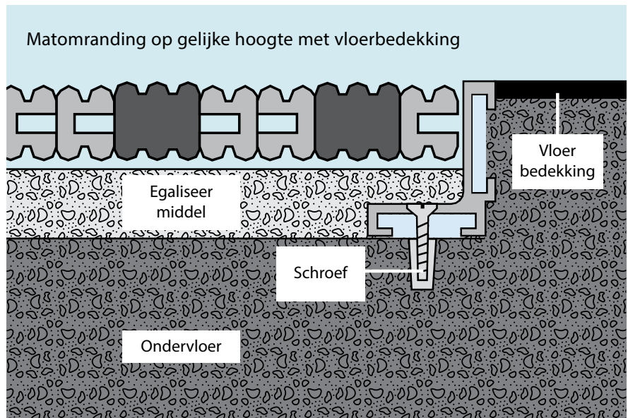
Doorsnede van een verzonken matomranding bevestigd met schroeven.
