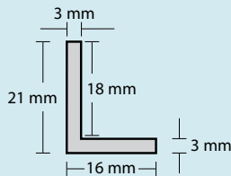
AMF 213
