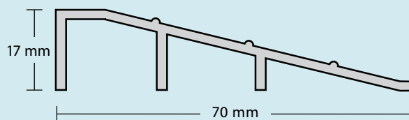
ARF 70
