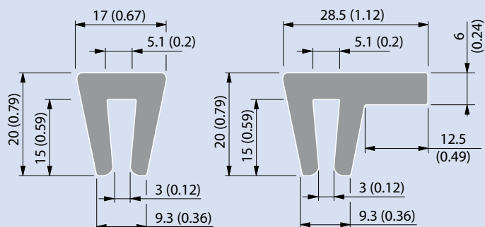
Tiras de desgaste extruidas
