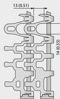
Variente dimensiones específicas [mm (in)]
