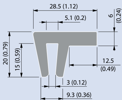
Tiras de desgaste extruidas
