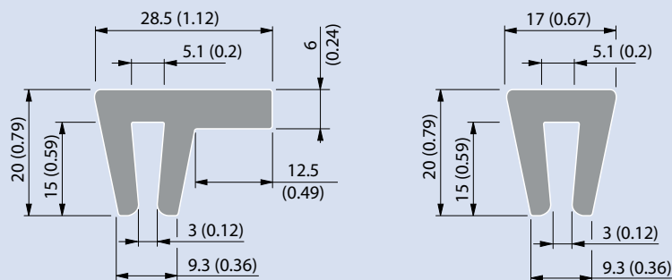
Tiras de desgaste extruidas
