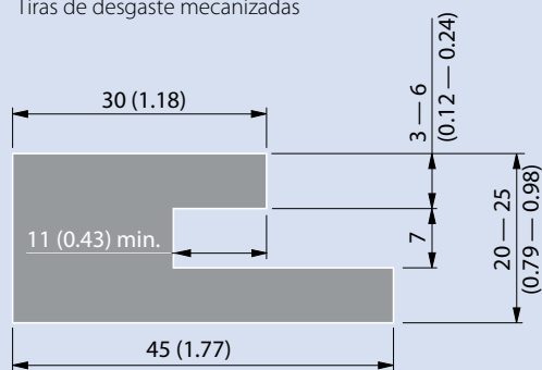
Tiras de desgaste mecanizadas
