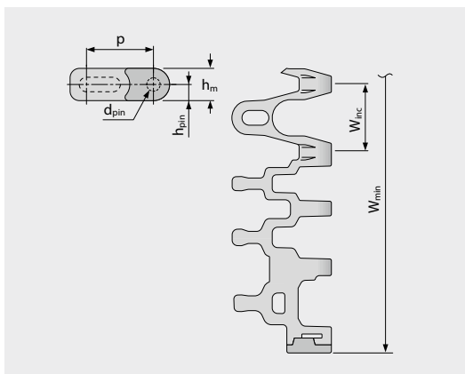
Variente dimensiones específicas [mm (in)]
