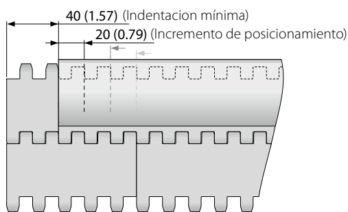
Configuración de indentacion S6.1-0 FLT PSU-0
