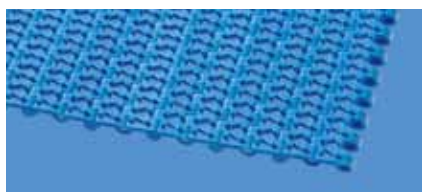
S4.1 | 21 % открыто | Пупырчатая поверхность
