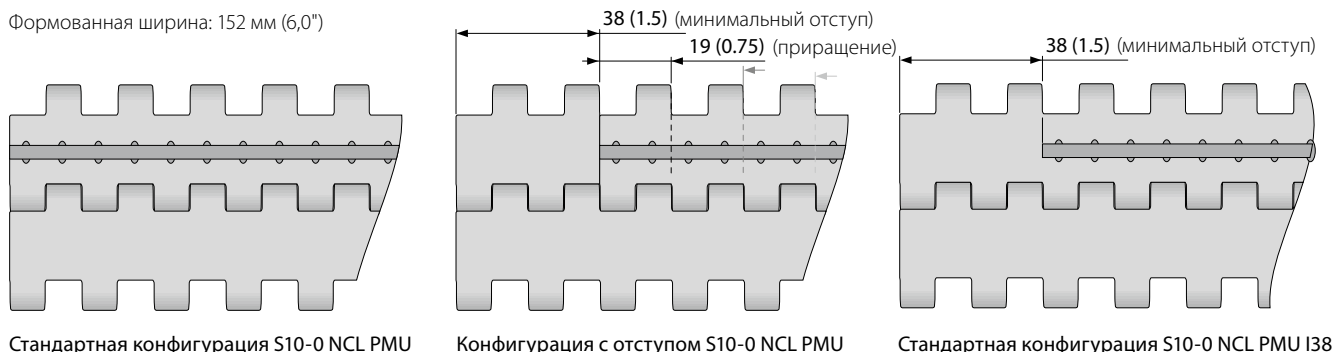
Стандартная конфигурация S10-0 NCL PMU
