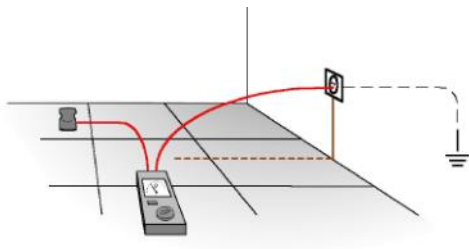
Schema doormeten van de vloer
