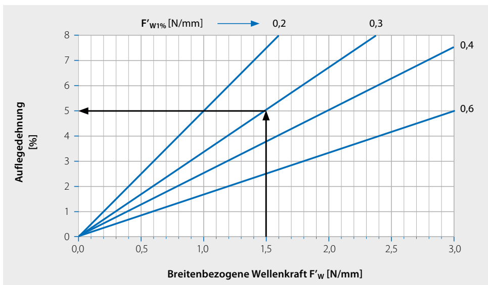
Diagramm 2: Ermittlung der Auflegedehnung
