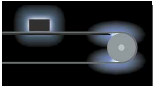
Elektrostatische Aufladung durch das Fördergut und durch den triboelektrischen Effekt.
