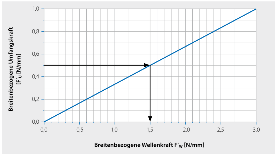
Diagramm 1: Ermittlung der Mindest-Wellenkraft
