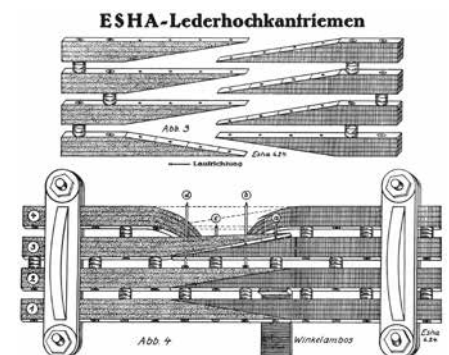
Oben: Aufbau des Chromleder-Hochkantriemens (Darstellung aus dem Jahr 1925).
