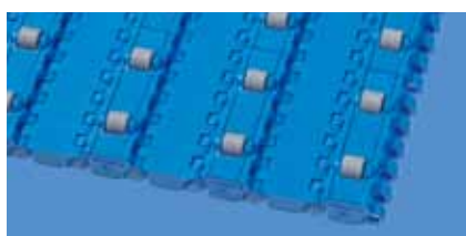
S8 | 0% open | Roller Top A90
