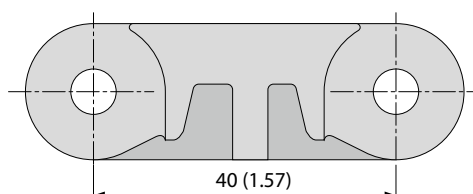
側面図 (比例1:1)
