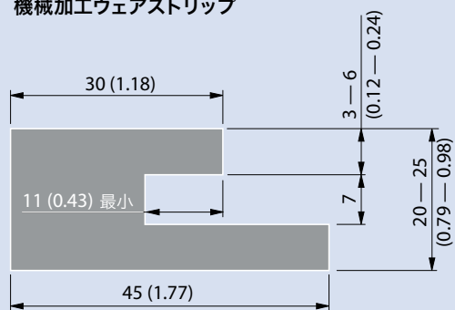
機械加工ウェアストリップ
