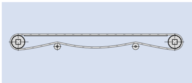
直進水平運動コンベヤ
