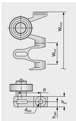
詳細寸法[ミリ (インチ)]
