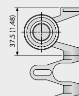
詳細寸法[ミリ (インチ)]
