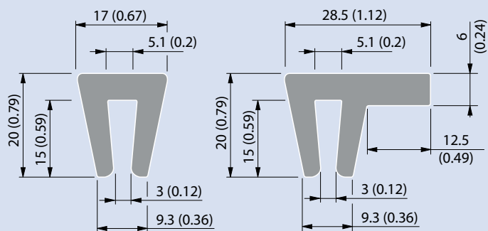
押出ウェアストリップ
