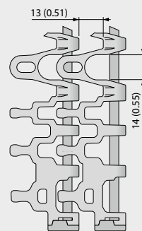
詳細寸法[ミリ (インチ)]
