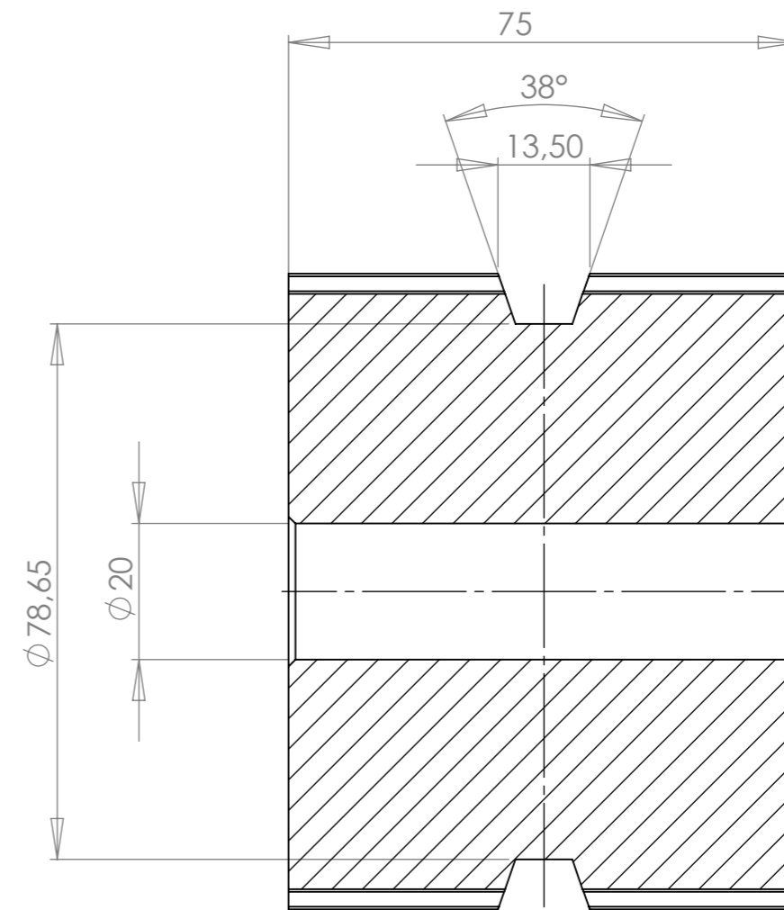
SCHNITT B-B MAßSTAB 1 : 1
